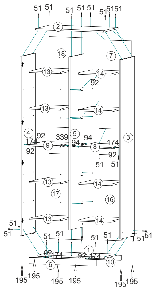
Сборка в левом исполнении
