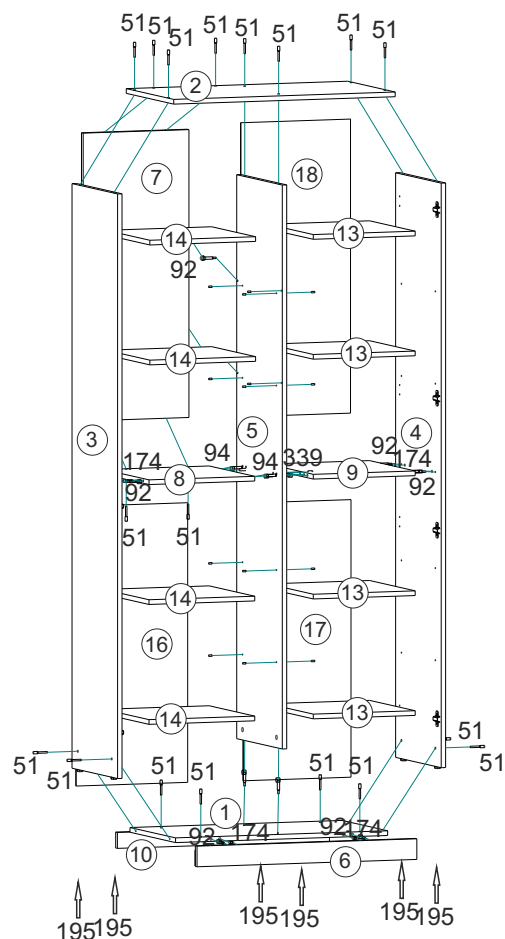
Сборка в правом исполнении
