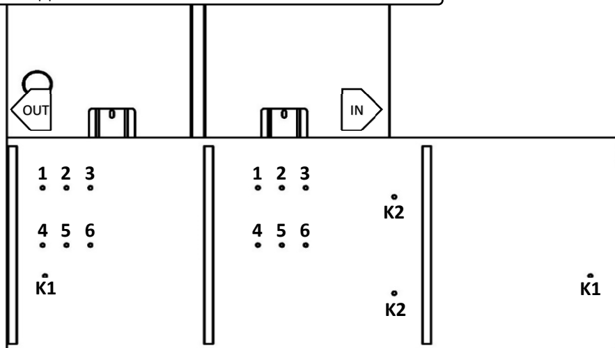
СХЕМА 2.1 - СВЕРЛЕНИЕ ОТВЕРСТИЙ В ВЕРХНЕЙ КРЫШКЕ ТУМБЫ
